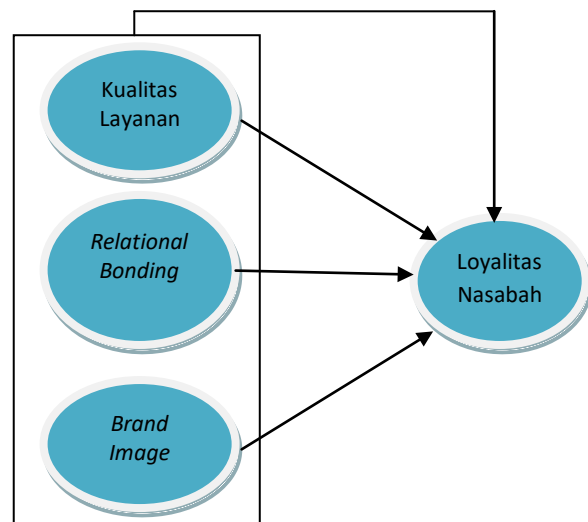
Gambar 1 Kerangka Konseptual
